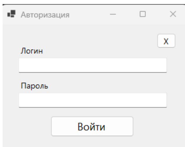
Рисунок 3.2 - Окно авторизации
