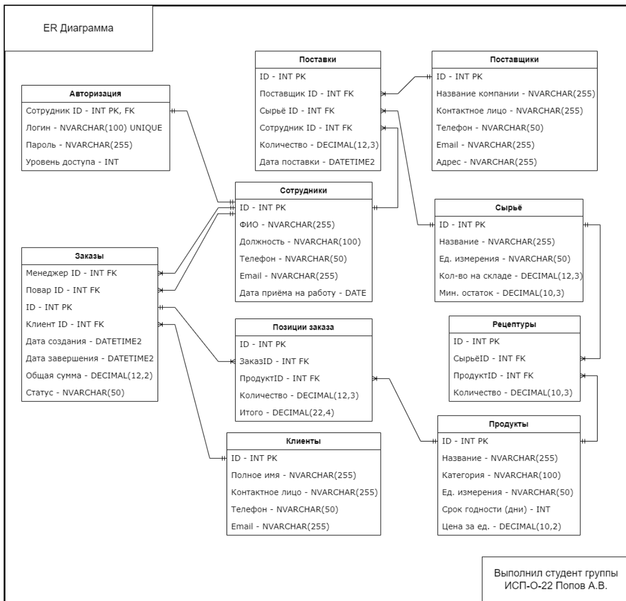
Рисунок 2.1 - ER Диаграмма
