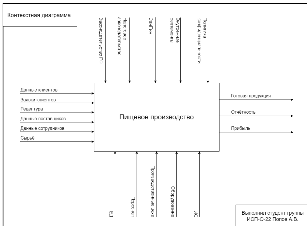
Рисунок 2.2 - Контекстная диаграмма
