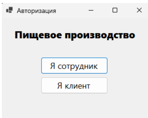
Рисунок 3.1 - Окно авторизации
